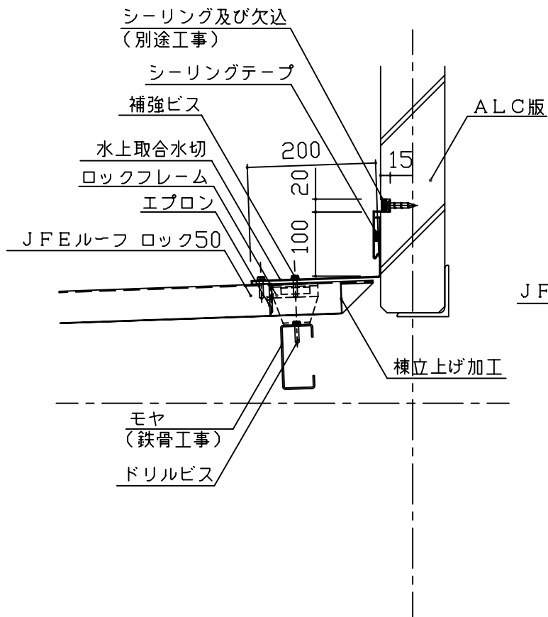
水上取合納まり図(1)
