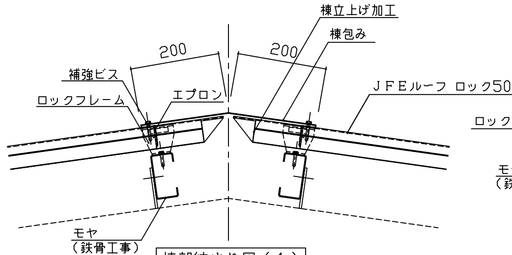
棟部納まり図(1)
