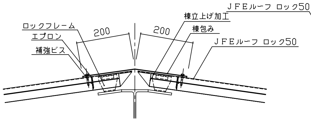
棟部納まり図(1)
