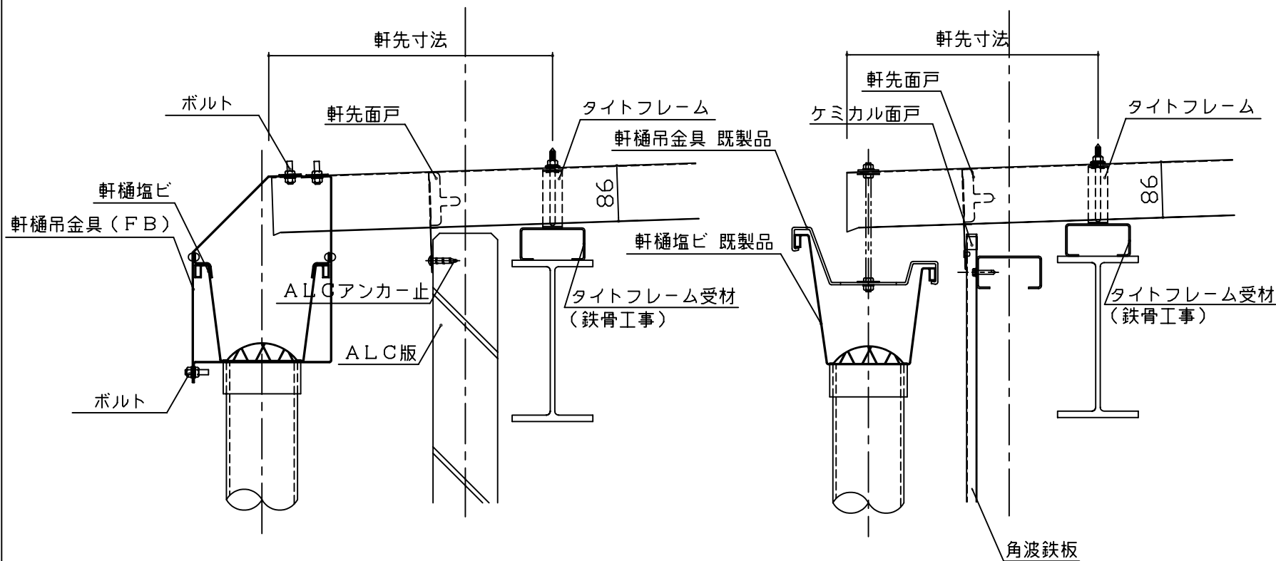
軒先納まり図(1)
