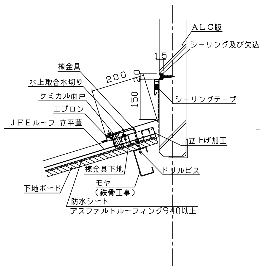
水上取合納まり図 (1)
