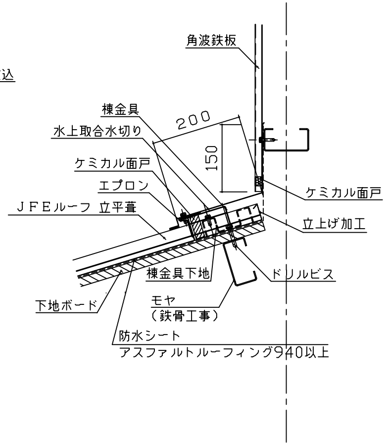
水上取合納まり図 (2)
