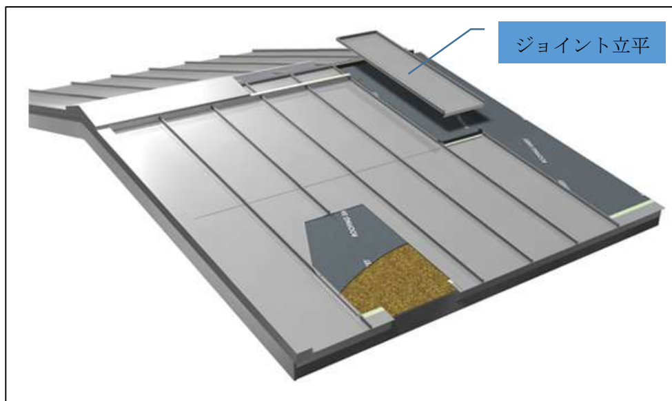
図 3 ジョイント立平概要図
