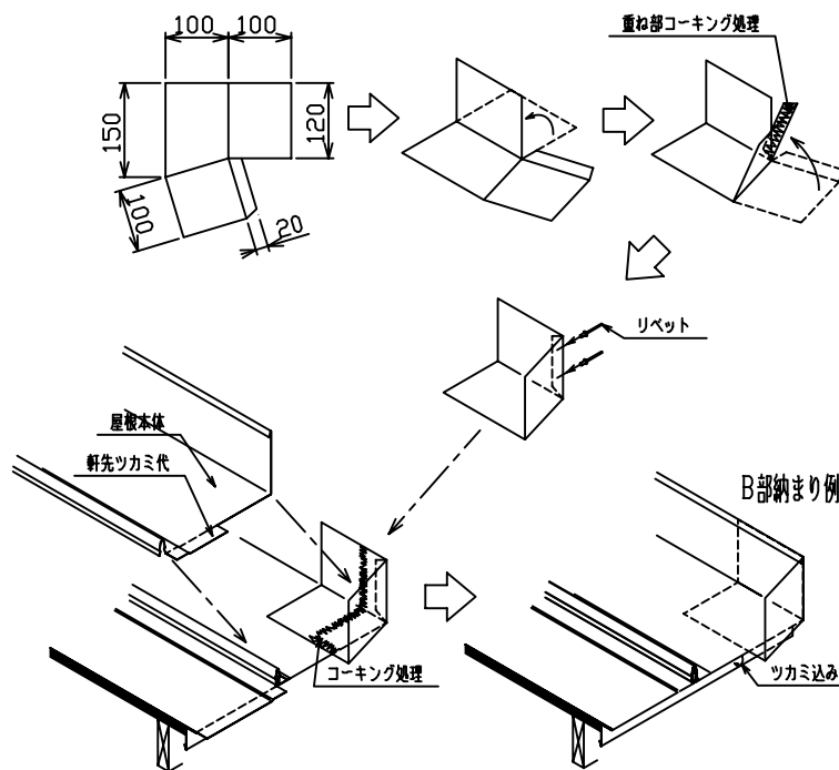
壁止まり役物加工例
