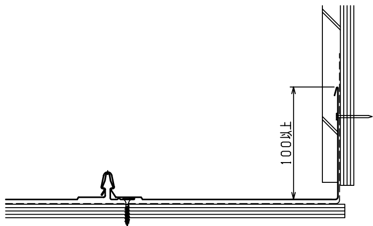
A-A' 断面図
